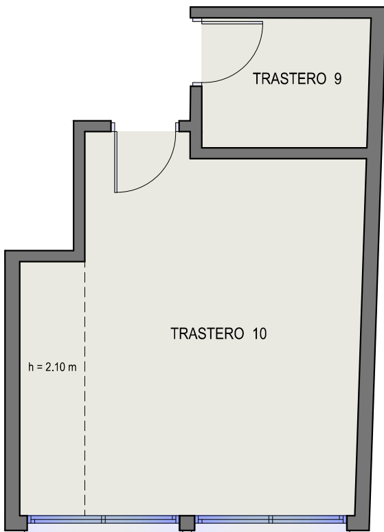
PLANTA SEMISÓTANO
