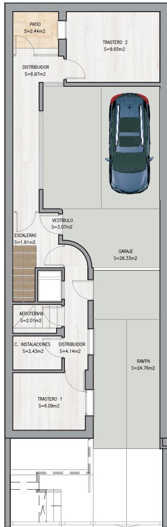
PLANTA SEMISÓTANO
